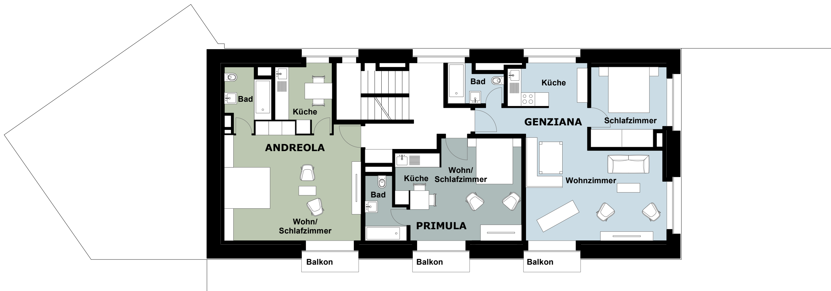
1. Obergeschoss
